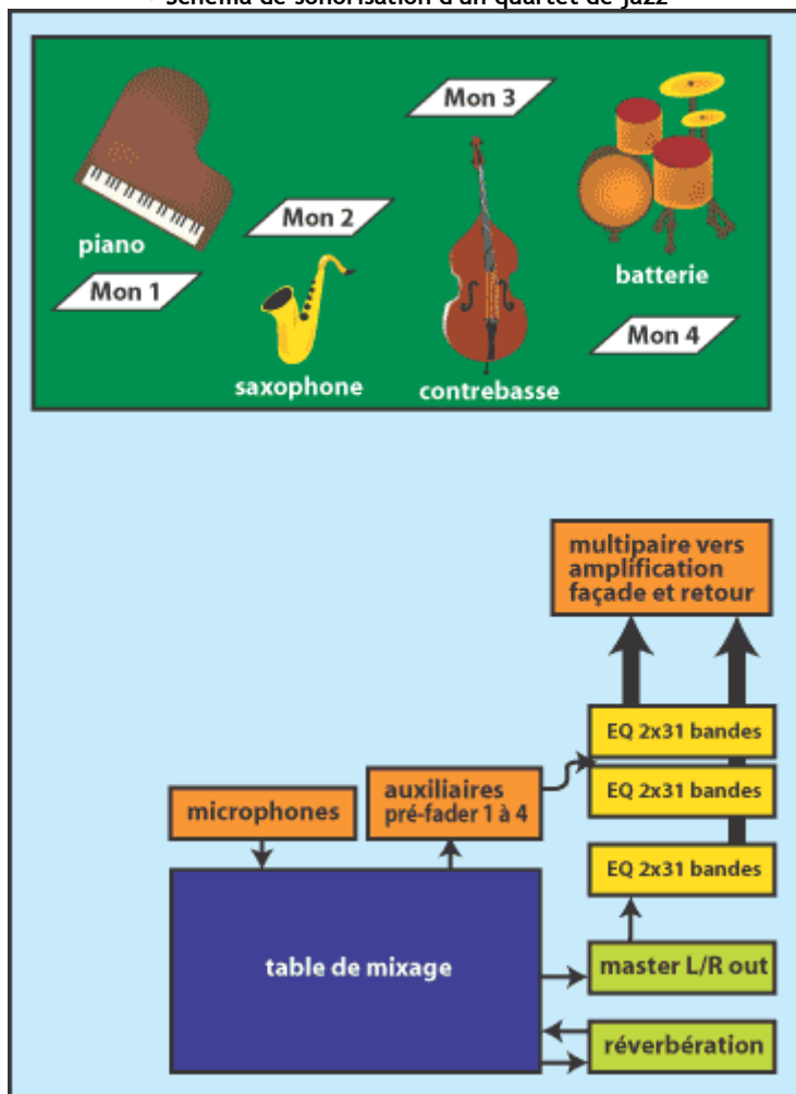
▼ Schéma de sonorisation d'un quartet de jazz
